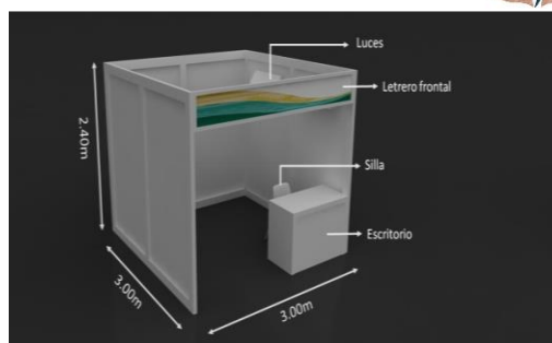
Stand Básico 2: 3m x 3m (9m 2 )
