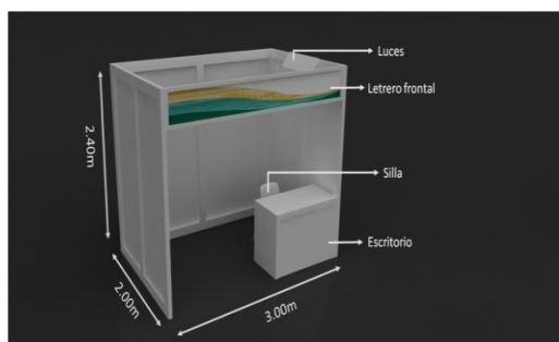
Stand Básico 1: 3m x 2m (6m 2 )
