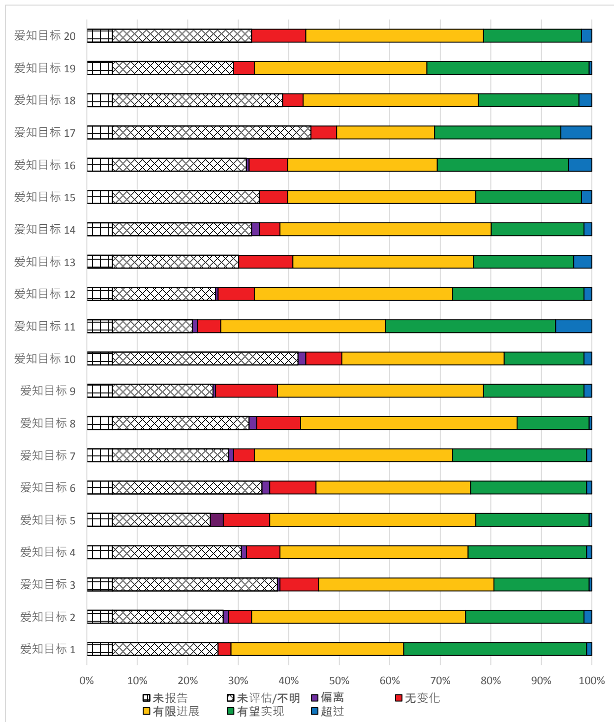
图 2. 根据第六次国家报告所报相应国家目标的进展情况对每项爱知生物多样性目标的进展的评估
