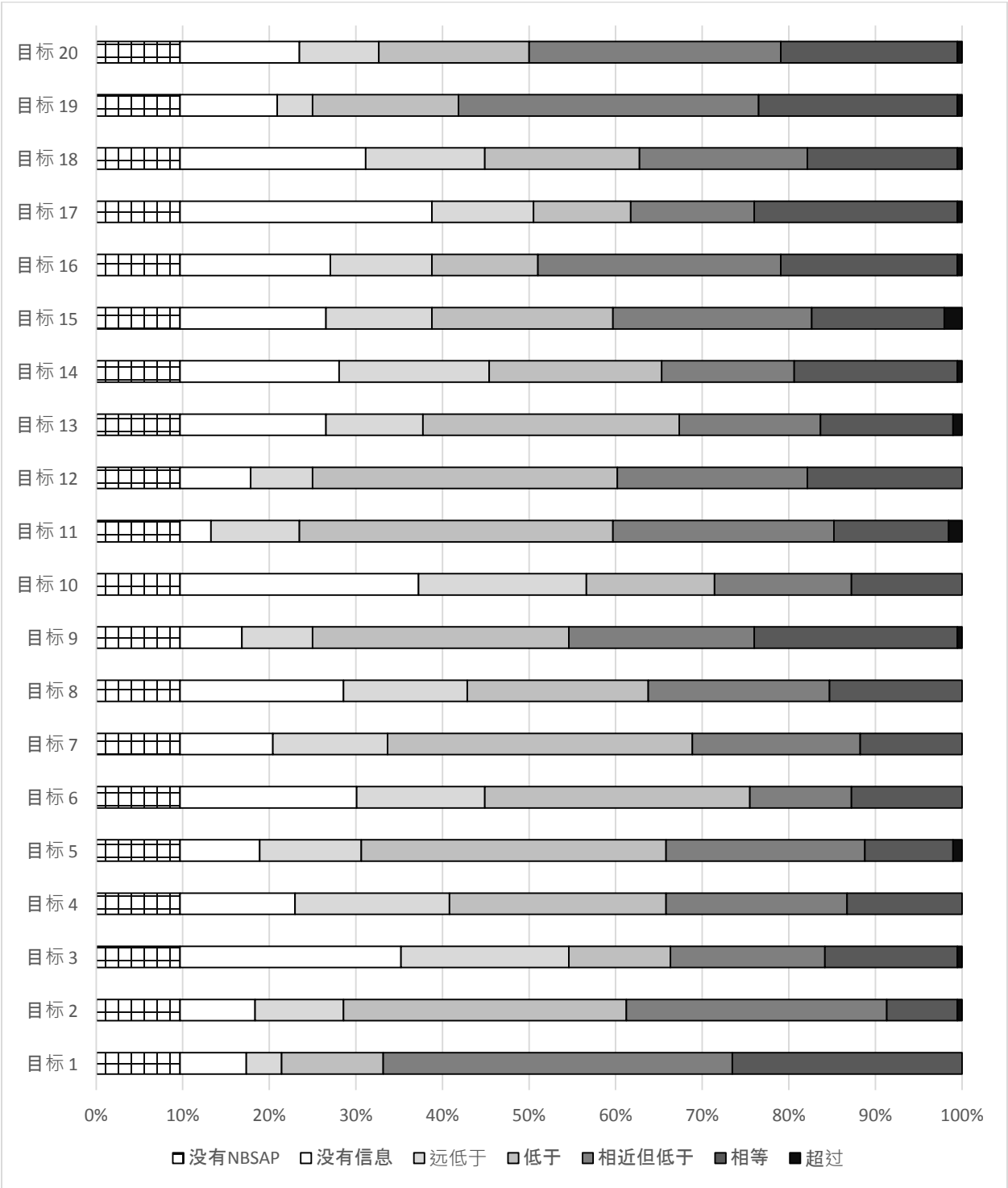
图 1. 对修订和更新版 NBSAP 中国家目标和其他承诺与爱知生物多样性目标的一致性的评估
