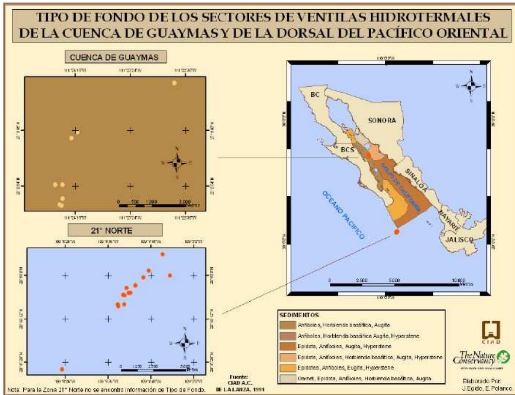
Figure 1. The geographic location of the Guaymas Basin. Image extracted from Comisión Nacional de Áreas Naturales Protegidas, 2006. “Estudio Previo Justificativo para el establecimiento del Santuario Ventiladas Hidrotermales de la Cuenca de Guaymas y de la Dorsal del Pacífico Oriental”. México, D.F., pp. 89 + anexos.
