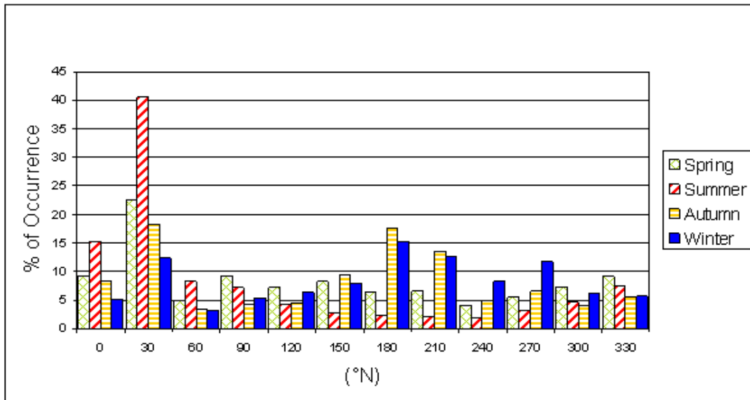
Figure 4. Distributions directionnelles saisonnières des courants supérieurs (Station 1).
