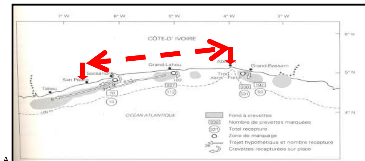
Figure 15. Importance écologique et biologique de l'aire marine de Tabou-Abidjan (Aire de répartition des crevettes roses dans les eaux marines côtières).
